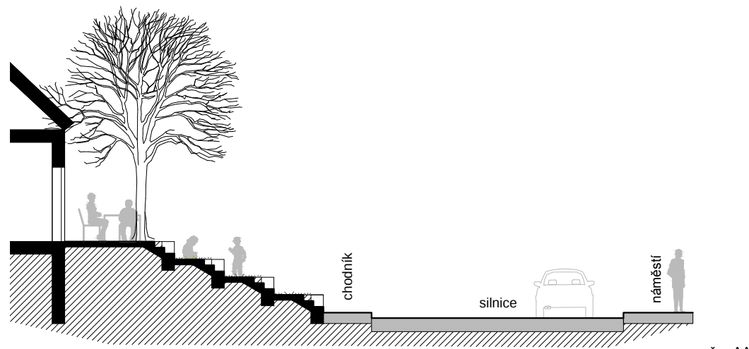
řez AA
