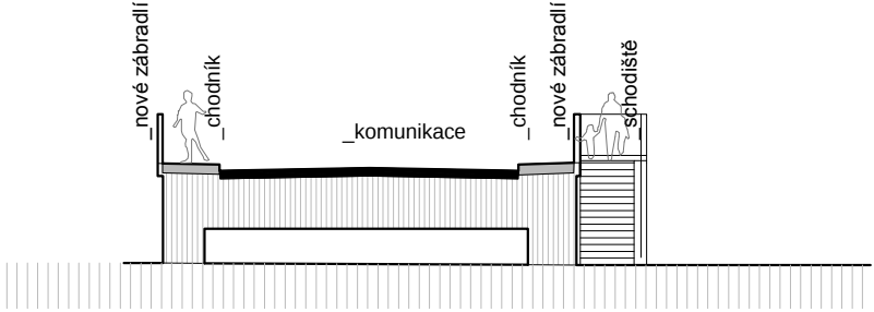
ŘEZ C-C'
