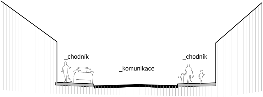
ŘEZ A-A'
