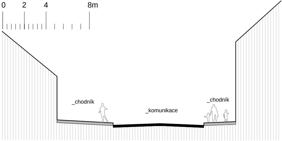
ŘEZ B-B'
